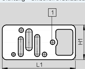
1 mit Bohrung, Steuerluftversorgung intern
